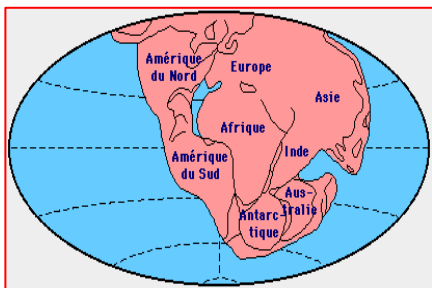
Pangée de Wegener
