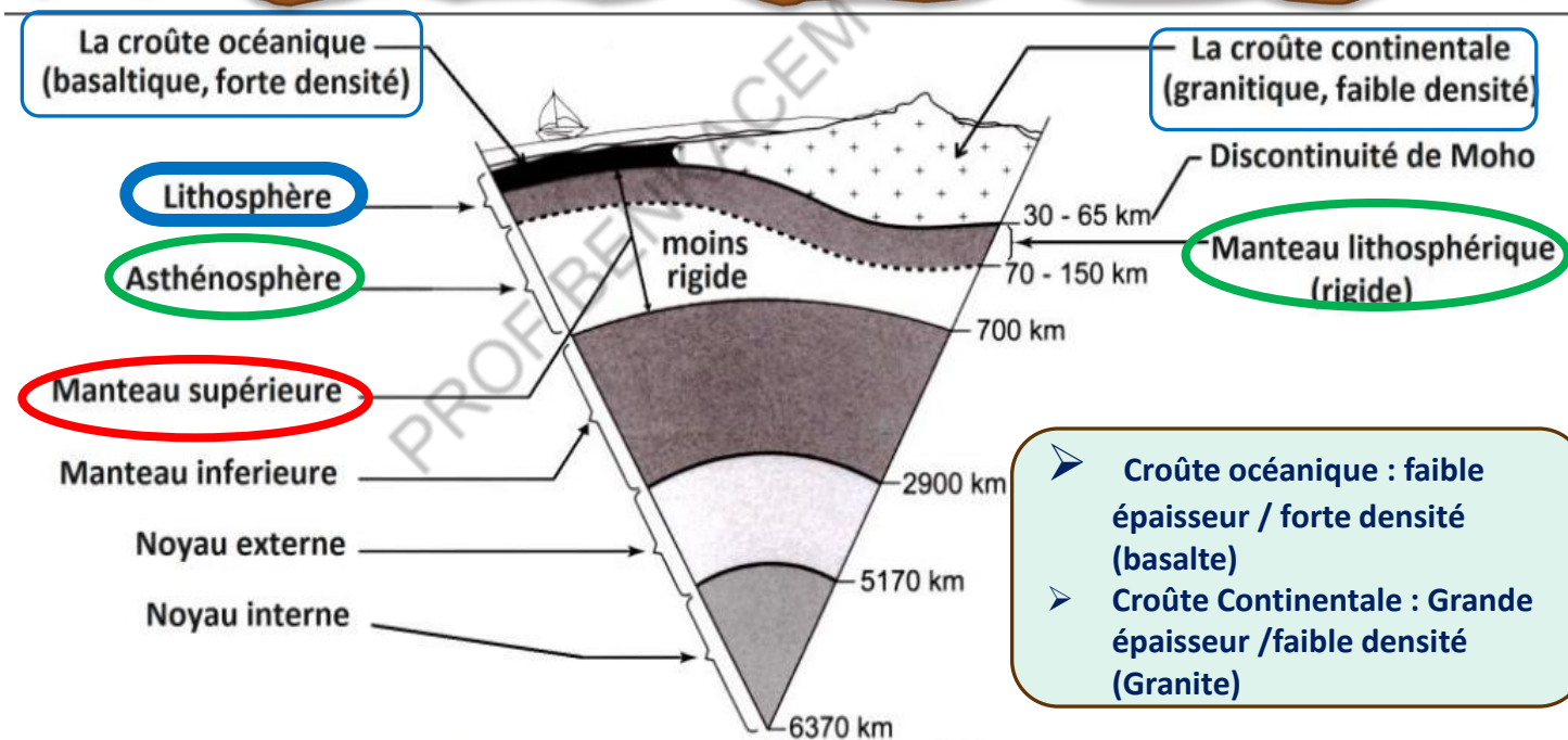
Fig 1. La structure interne du globe terrestre
